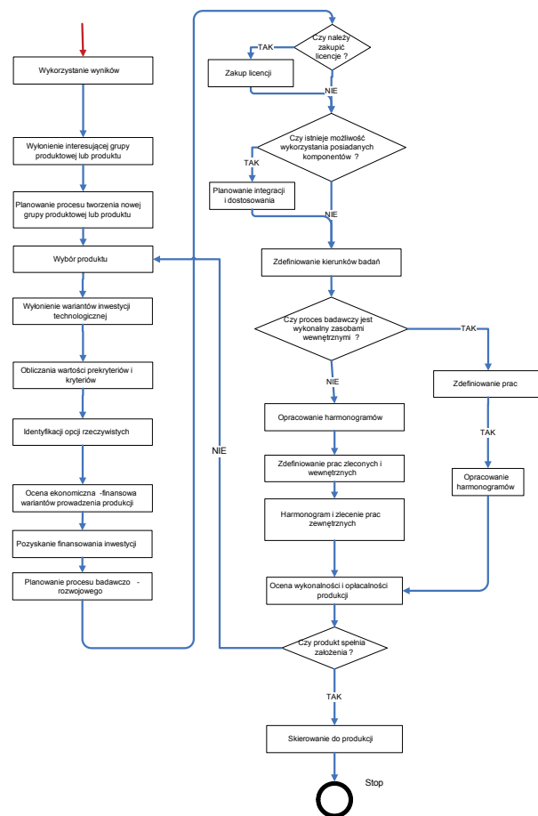
Rys. 1. Schemat rozwiązywania technologicznych problemów decyzyjnych metodą roadmappingu
